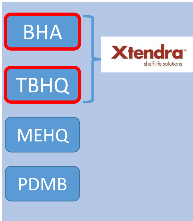
Idrochinone
