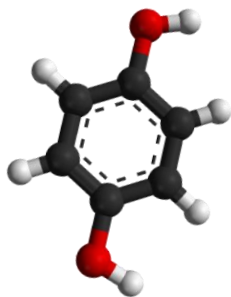
Idrochinone
