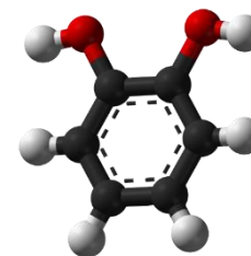
Catecolo
